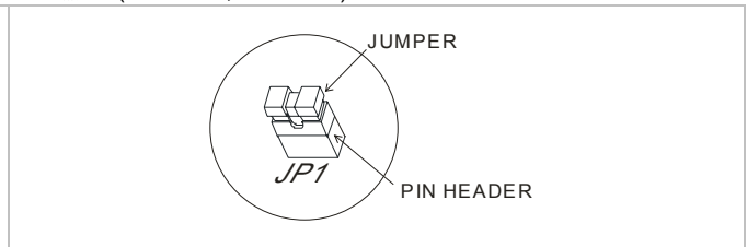
電流輸入（4 ~ 20mA, 0 ~ 20mA）
